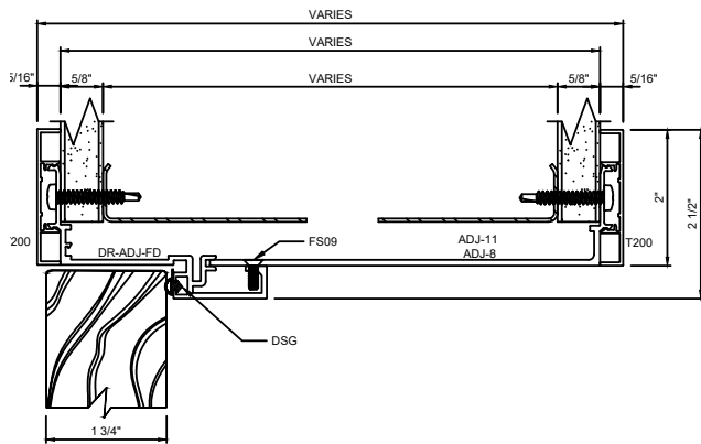
A DOOR FRAME HEADER
