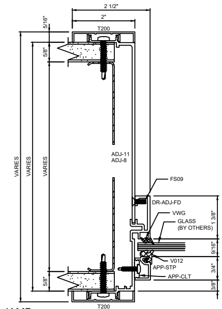
C DOOR FRAME STRIKE JAMB
