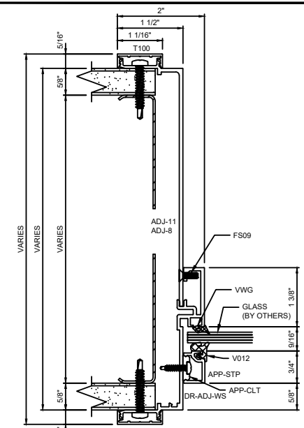
C DOOR FRAME STRIKE JAMB
