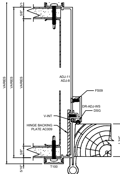
B DOOR FRAME HINGE JAMB
