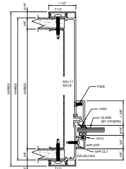
C DOOR FRAME STRIKE JAMB
