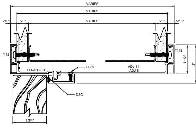
A DOOR FRAME HEADER
