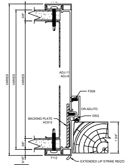
C DOOR FRAME STRIKE JAMB
