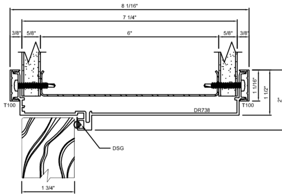
A DOOR FRAME HEADER
