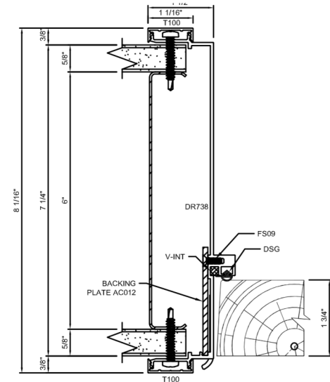
C DOOR FRAME STRIKE JAMB
