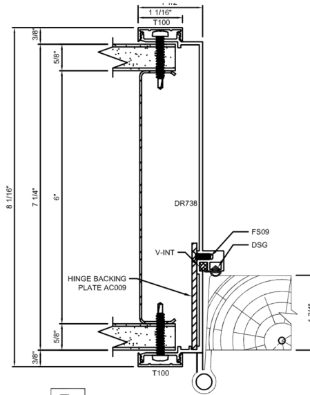
B DOOR FRAME HINGE JAMB
