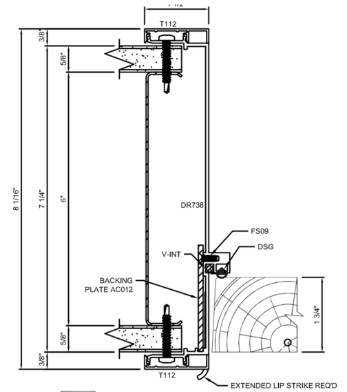
C DOOR FRAME STRIKE JAMB
