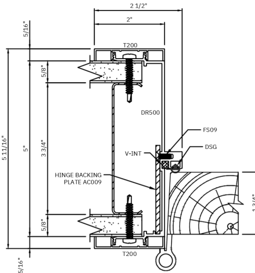
B DOOR FRAME HINGE JAMB
