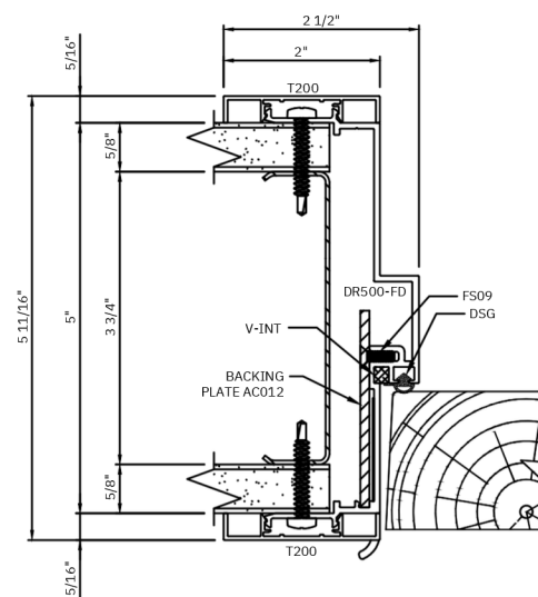
C DOOR FRAME STRIKE JAMB
