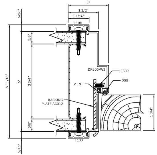
C DOOR FRAME STRIKE JAMB
